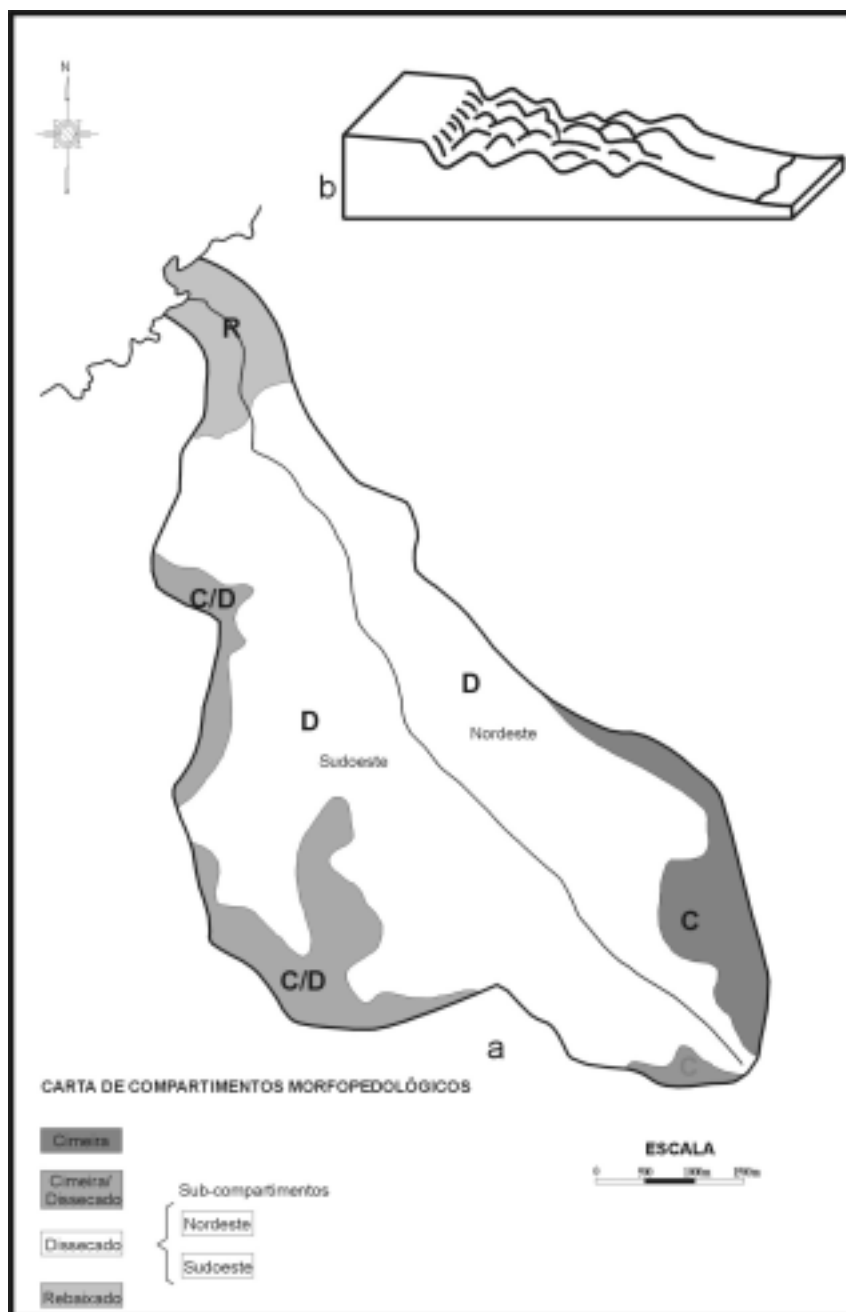
Figura 7 – Compartimentos morfopedológicos vistos em planta (a), e em bloco-diagrama (b)
