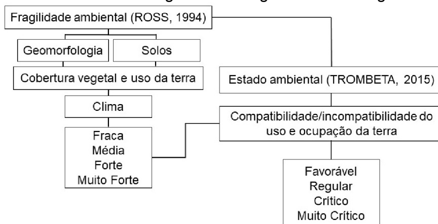
Figura 2. Fluxograma metodológico.
